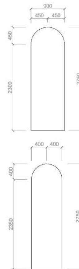
Kích thước ô chò tiêu chuẩn
