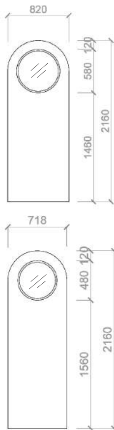
Kích thước ô kính trên cánh tiêu chuẩn
