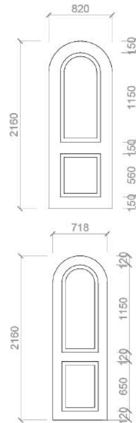
Kích thước phào trên cánh tiêu chuẩn
